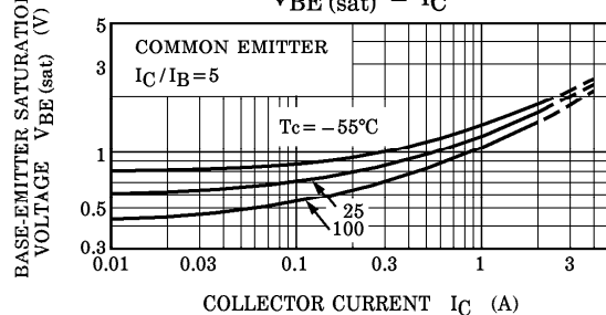
V_{BE(sat)} - I_C
