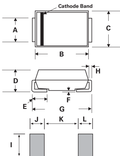
DO-214AA (SMB J-Bend)
