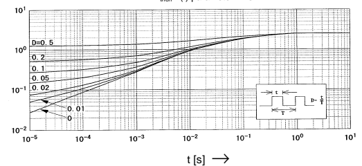
Transient Thermal Impedance Z_{th(ch-e)}=f(t) parameter: D=t/T
