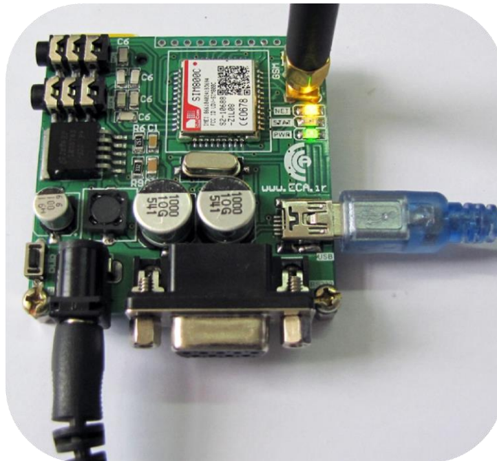
در صورت عدم وجود درگاه RS232 در کامپیوتر می توان از USB به سریال برد استفاده کرد.
