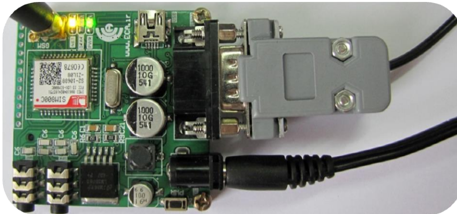
در صورت عدم وجود درگاه RS232 در کامپیوتر می توان از USB به سریال برد استفاده کرد.
