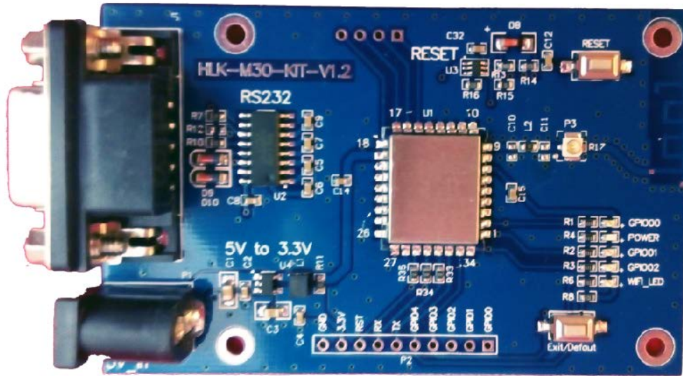
HLK-M30 StartKit
